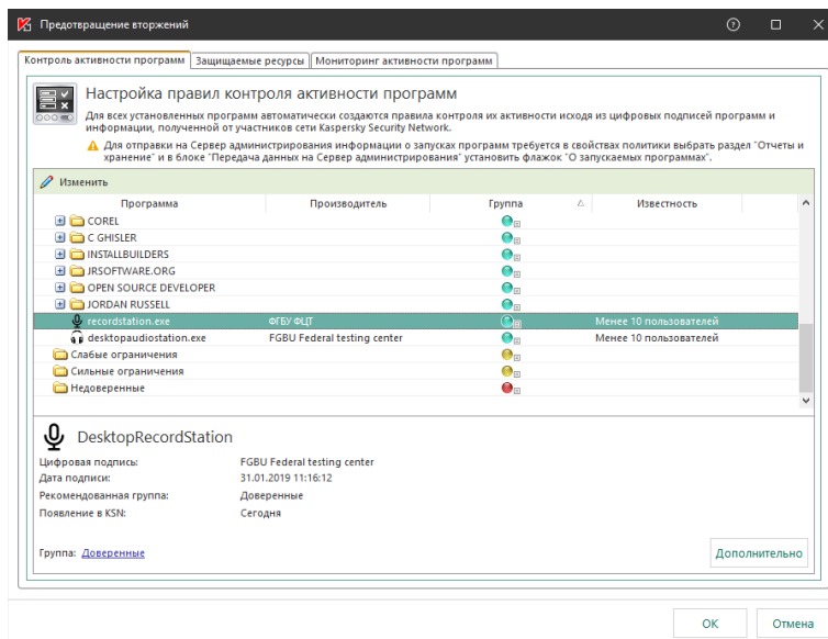
Рис. 45. Kaspersky Endpoint Security для Windows. Применить настройки
