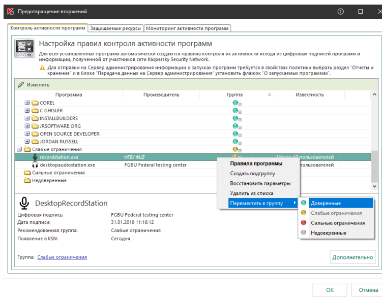
Рис. 44. Kaspersky Endpoint Security для Windows. Настройка правил контроля активных программ
