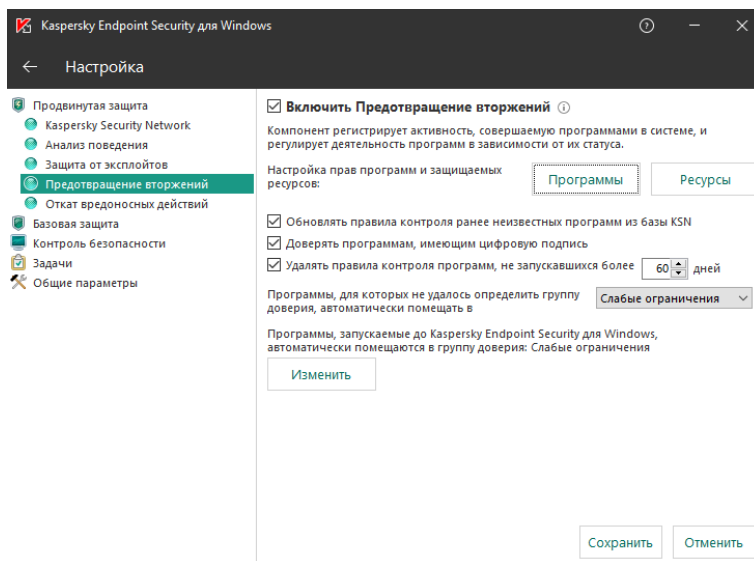
Рис. 46. Kaspersky Endpoint Security для Windows. Сохранить настройки
